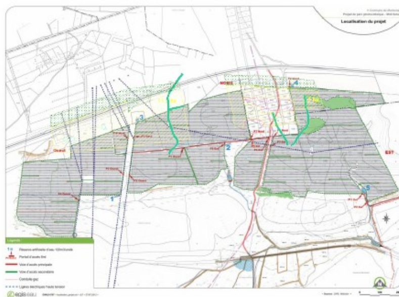
Plan d'implantation général de la ferme photovoltaïque en 2011 et localisation du projet 2016 Tamareau Solar 1 (jaune et vert)
